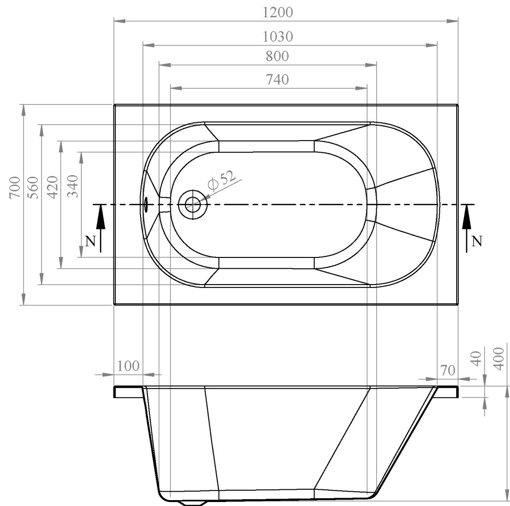
PRZEKRÓJ N-N SKALA 1 : 13
